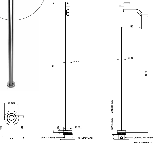
Miscelatore lavabo a pavimento Floor basin mixer column
