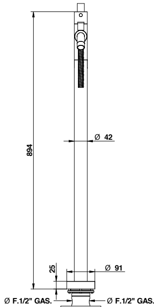
Miscelatore vasca a pavimento con set doccia e deviatore Bath mixer to the floor with shower set and diverter
